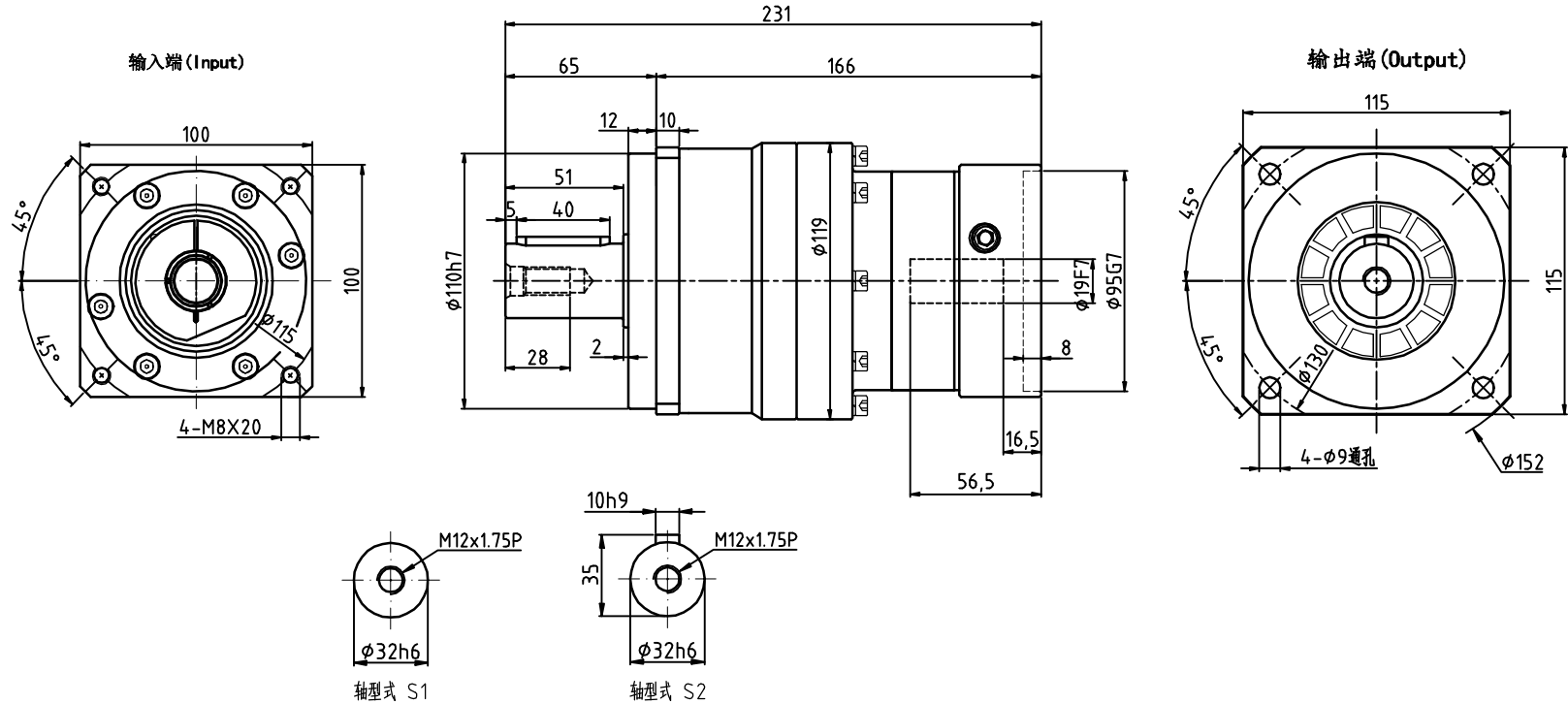
尺寸图
