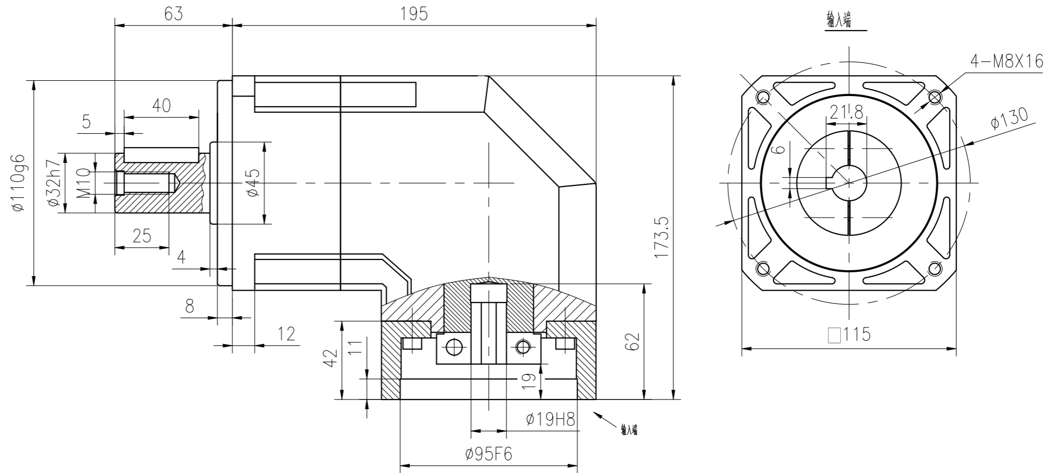
PGR115 单级 参数表 Parameters
