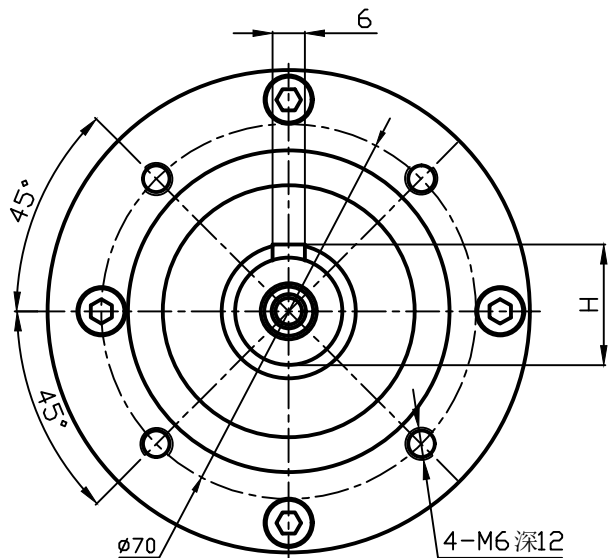
输出端(output)
